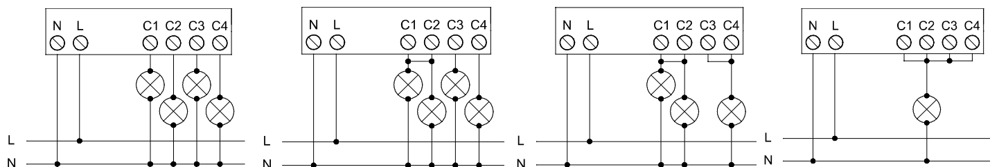
Σχήμα 2: Παραδείγματα συνδεσμολογίας (από αριστερά προς τα δεξιά):
