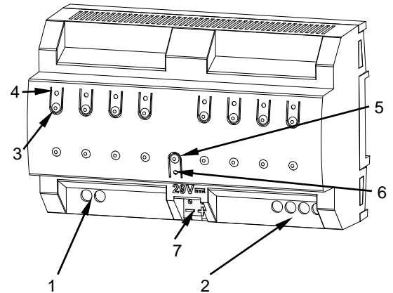
Σχήμα 1: DIMinBOX DX4
