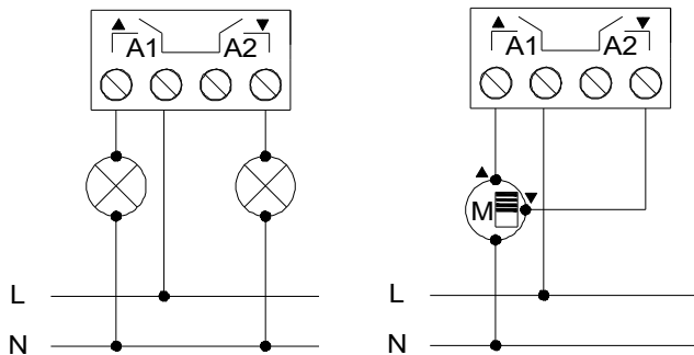
Σχήμα 2. Παραδείγματα συνδεσμολογίας (από αριστερά προς τα δεξιά): 2 ανεξάρτητα φορτία και 1 κανάλι ρολών/περσίδων.
