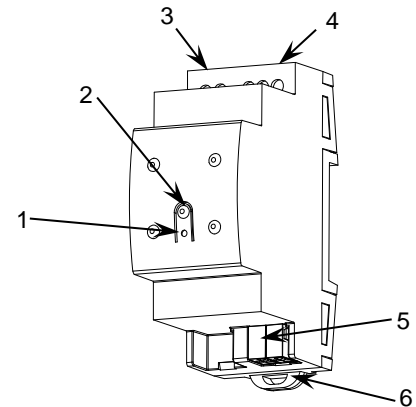
Figura 1: KLIC-DI v2
