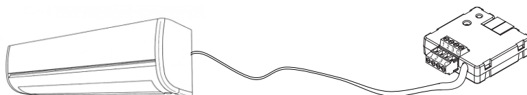
Figure 2. Câblage du KLIC-MITT à machine Mitsubishi
