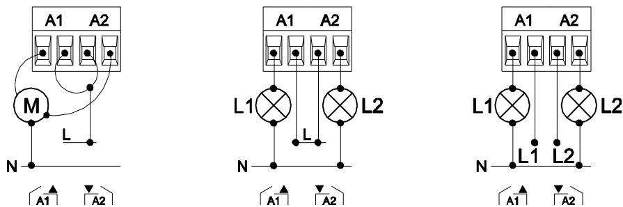
Figura 2. Ejemplos de conexiones (de izquierda a derecha): canal A como canal persiana y como salidas individuales con la misma y con diferentes fases.
