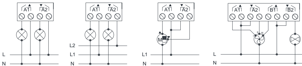
Figura 2: Ejemplo de conexionado (de izquierda a derecha): 2 cargas, 2 cargas a fases distintas, persiana y fan coil
