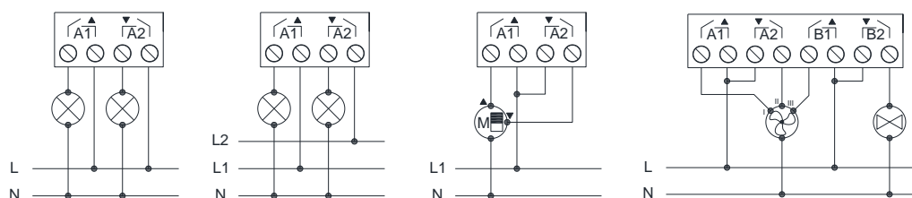
Figure 2: Exemples de connexions (de gauche à droite): 2 charges, 2 charges a phases différentes, volet roulant et ventilateur convecteur Fixer le MAXinBOX 24 v2 sur le rail DIN:
