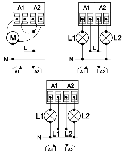
Σχήμα 2: (Από πάνω προς τα κάτω και από αριστερά προς τα δεξιά) Παραδείγματα συνδεσμολογίας για ρολό/περσίδα, ρελέ με ίδια φάση ή ρελέ με διαφορετικές φάσεις.
