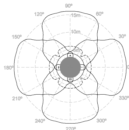
Σχήμα 2. Εύρος ανίχνευσης παρουσίας και κίνησης.
