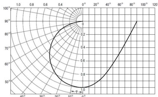
Σχήμα 4. Ευαισθησία αισθητήριου φωτεινότητας.
