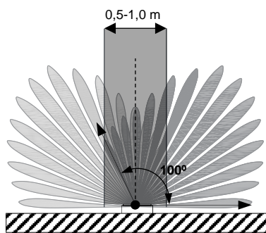
Figura 3: Sectores de detección (vista superior)
