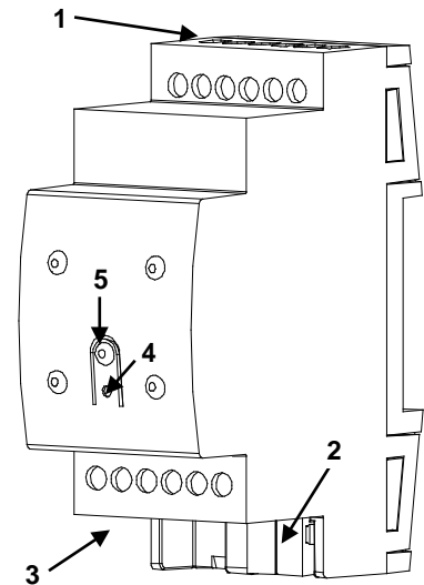
Рисунок 1: RailQUAD 8
