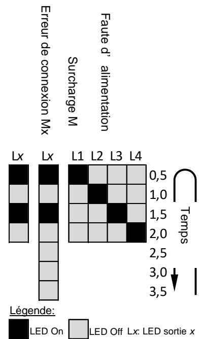
Figure 2: Notification d'erreurs au moyen de LED d'état de grille
