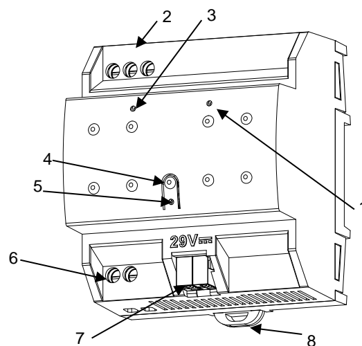
Figura 1: Fuente de alimentación ZPS320HIC110
