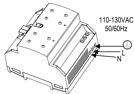
Figura 2: Instalación y conexión ZPS320HIC110
