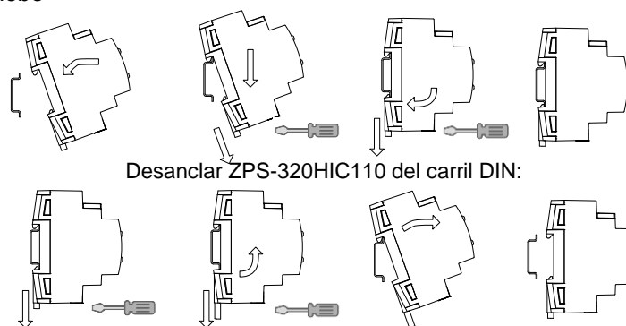
Figura 2: Instalación y conexión ZPS320HIC110
