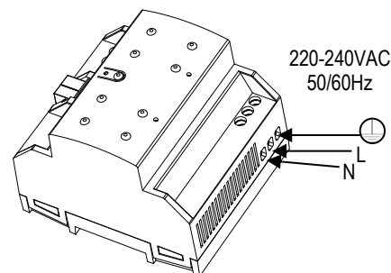
Figura 2: Instalación y conexión ZPS640HIC230
