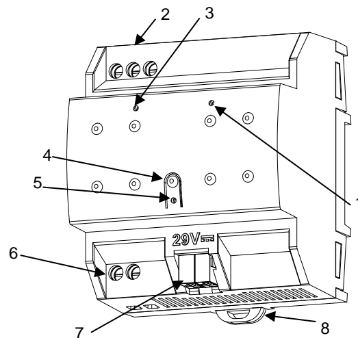
Figura 1: Fuente de alimentación ZPS640HIC230
