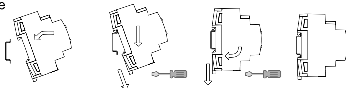
Figura 2: Instalación y conexión ZPS640HIC230
