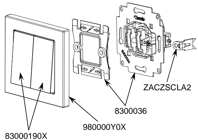
Figura 1. Pulsador doble
