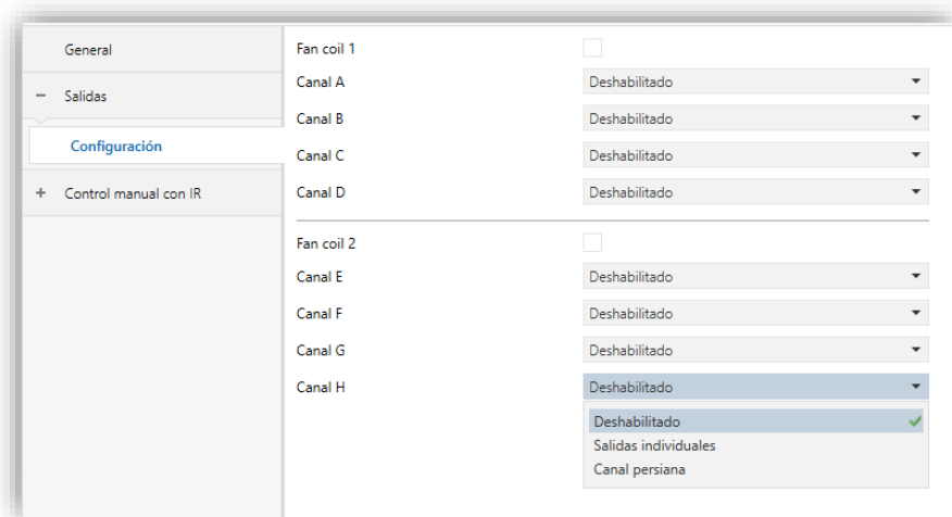
Figura 11. Pestaña salidas.
