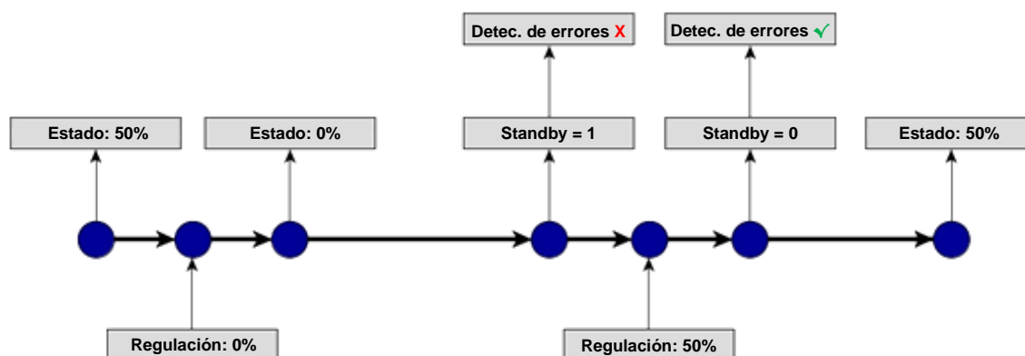
Figura 18. Secuencia de acciones ante Modo Standby
