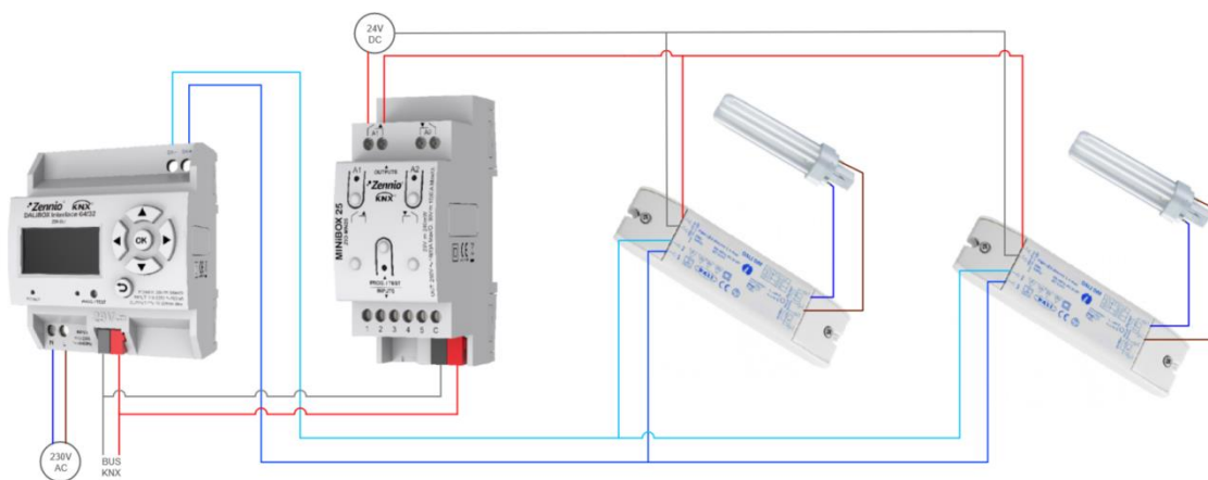
Figura 17. Sugerencia de conexionado para la función de Standby
