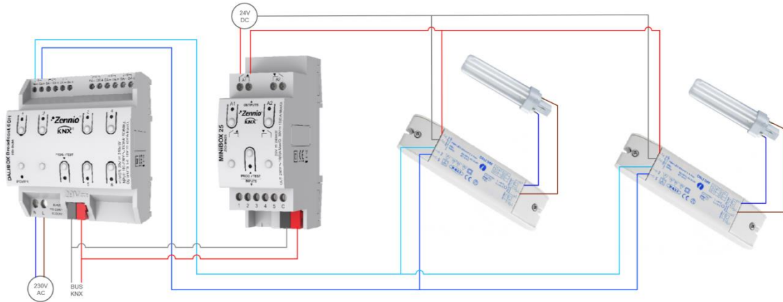
Figura 22. Esquema de funcionalidad Standby
