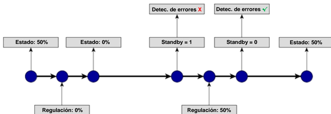
Figura 23. Secuencia de acciones ante Modo Standby
