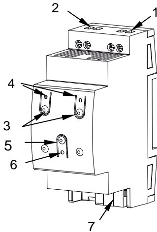
Figura 3 DIMinBOX DX1 – Diagrama de elementos
