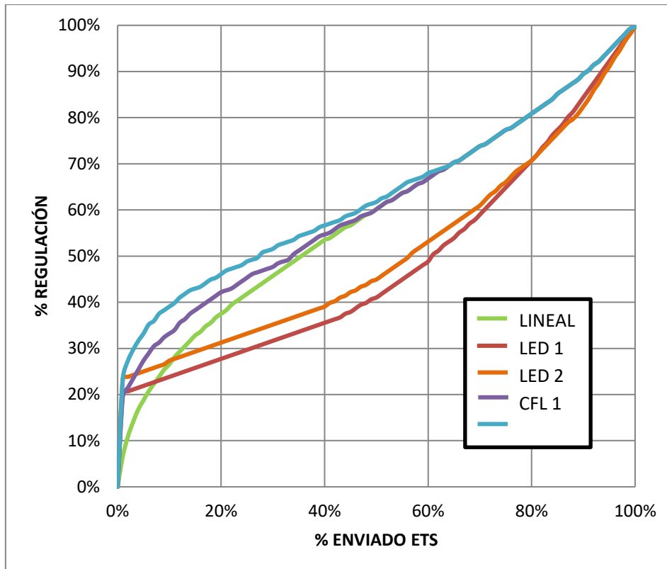
Figura 10 Curvas de regulación para cargas led y CFL.
