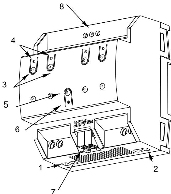
Figura 4 DIMinBOX DX2 – Diagrama de elementos.
