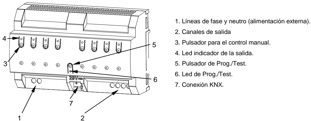
Figura 5 DIMinBOX DX4 – Diagrama de elementos.
