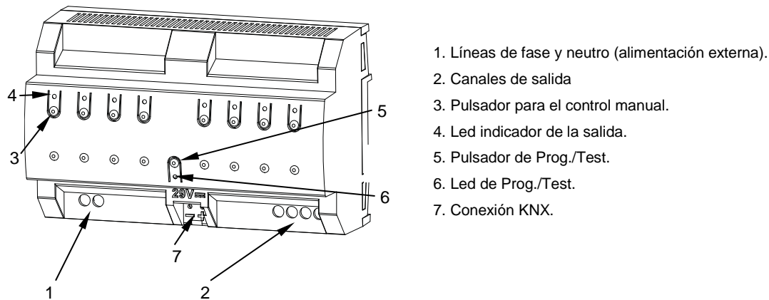
Figura 5 DIMinBOX DX4 – Diagrama de elementos.
