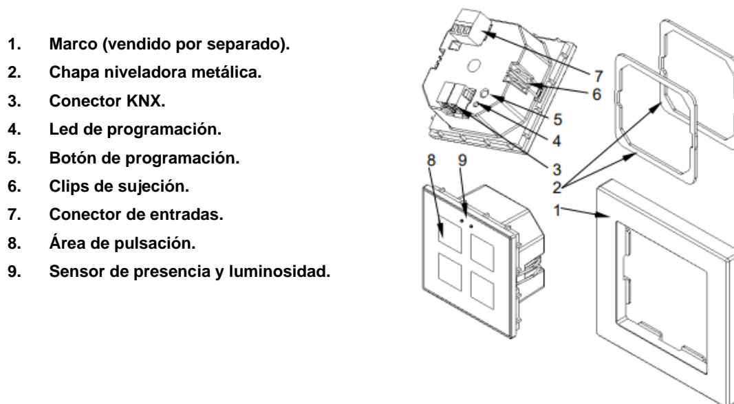
Figura 2 Diagrama de elementos Flat 55 v2
