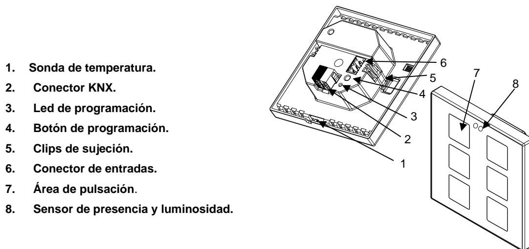
Figura 1 Diagrama de elementos Flat v2.
