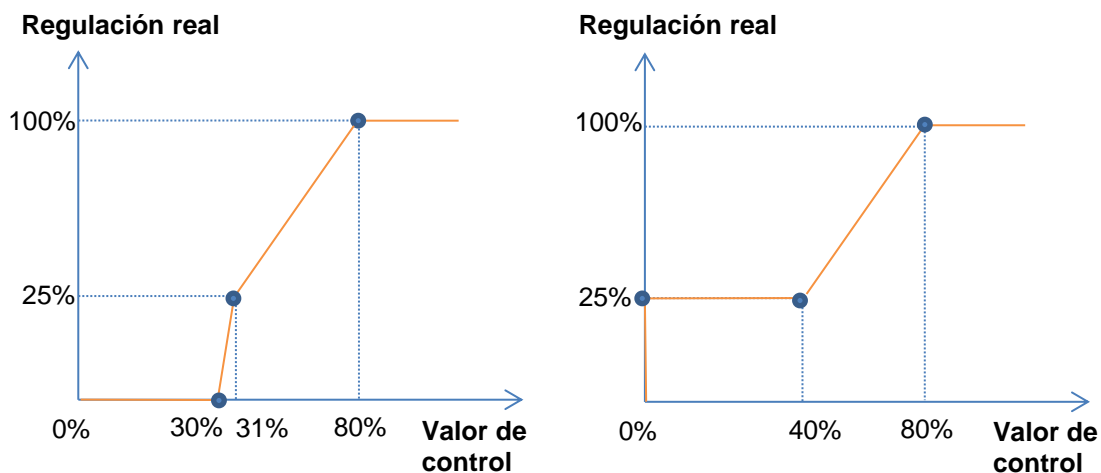
Figura 13 Curvas de control personalizadas.
