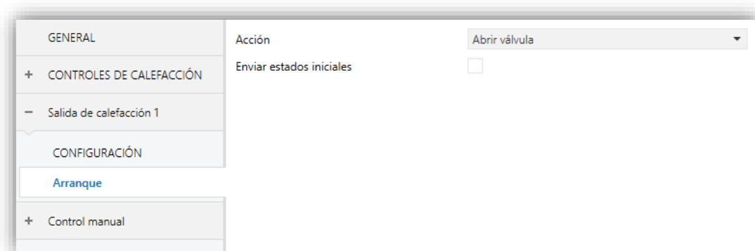
Figura 11 Control de calefacción - Arranque.
