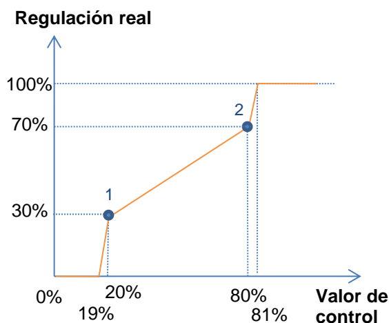
Figura 14 Curva característica - Valores fuera de rango.
