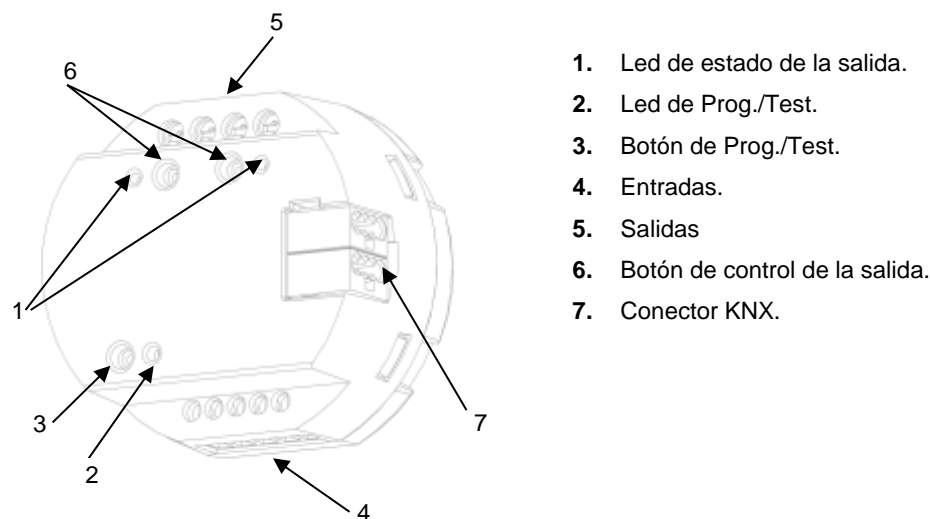
Figura 1. inBOX 24. Elementos.
