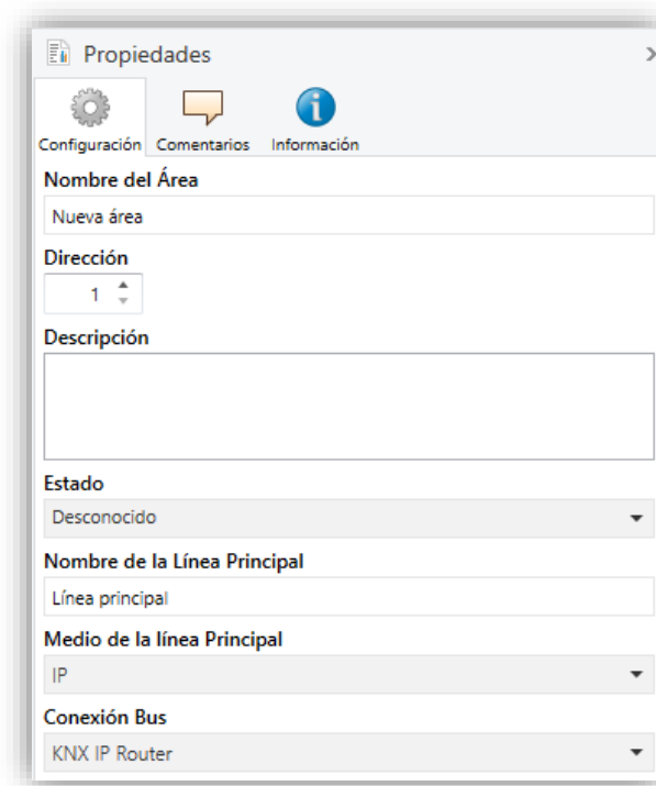
Figura 3 Captura de ETS5 para programación en paralelo.
