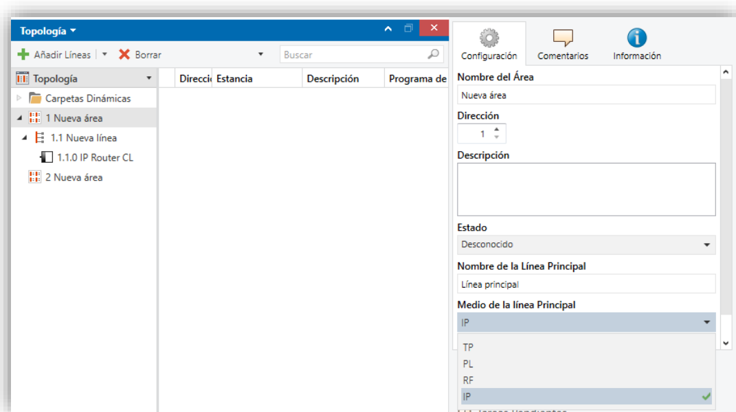
Figura 15 IP Router CL como acoplador de líneas.
