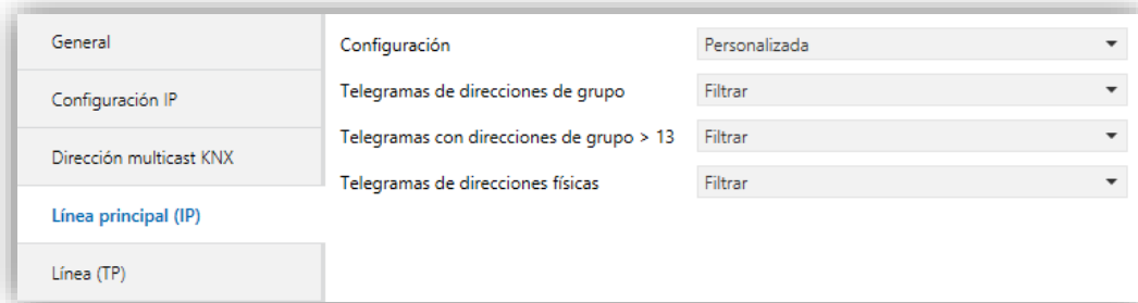
Figura 19 Pestaña de configuración de la línea principal (IP)
