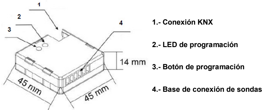
Figura 2. KES. Esquema de elementos.
