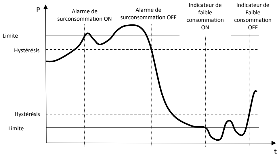
Figure 5. Supervision des limites de puissance
