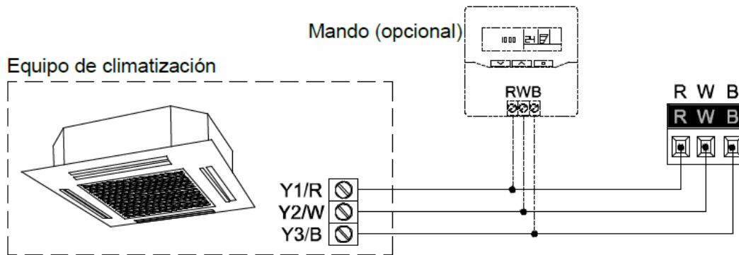
Figura 2. Conexión del KLIC-FJ vT a la máquina de A/A.
