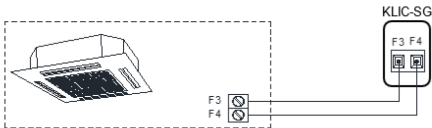
Figure 2. Connexion du KLIC-SG vT au bus F3/F4
