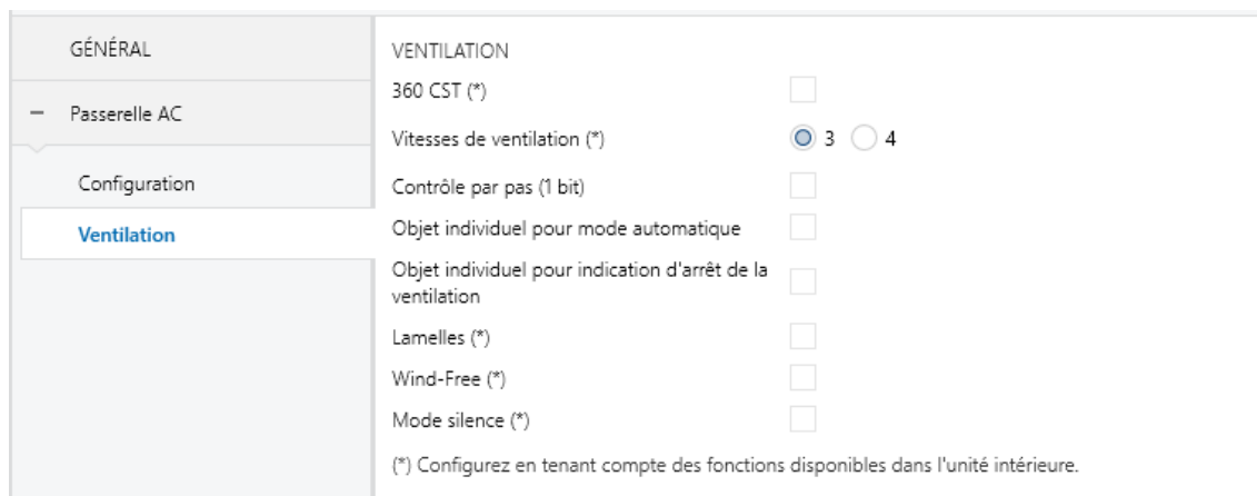
Figure 18. Passerelle d'A/C. Ventilateur
