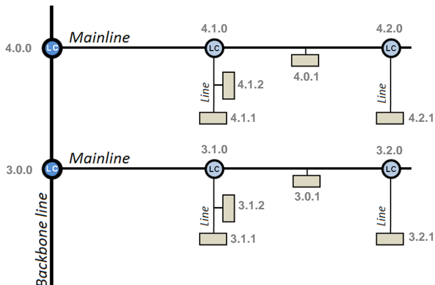
Figura 4 Acoplamiento de líneas
