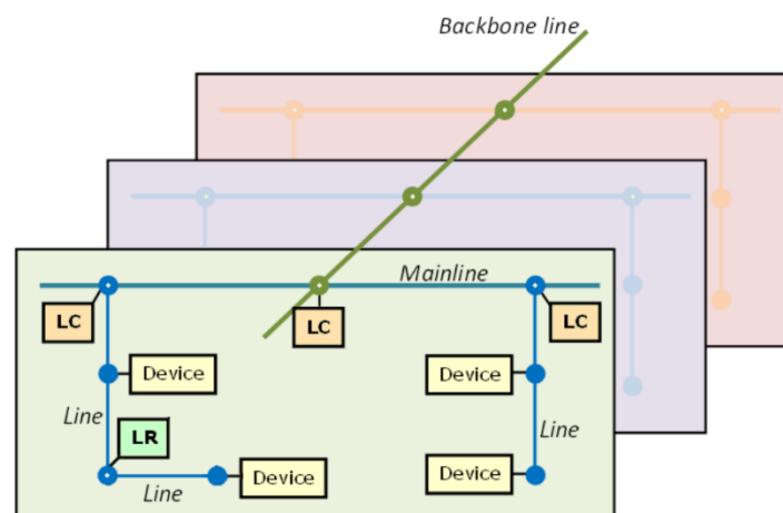
Figura 2 Contexto (topología)
