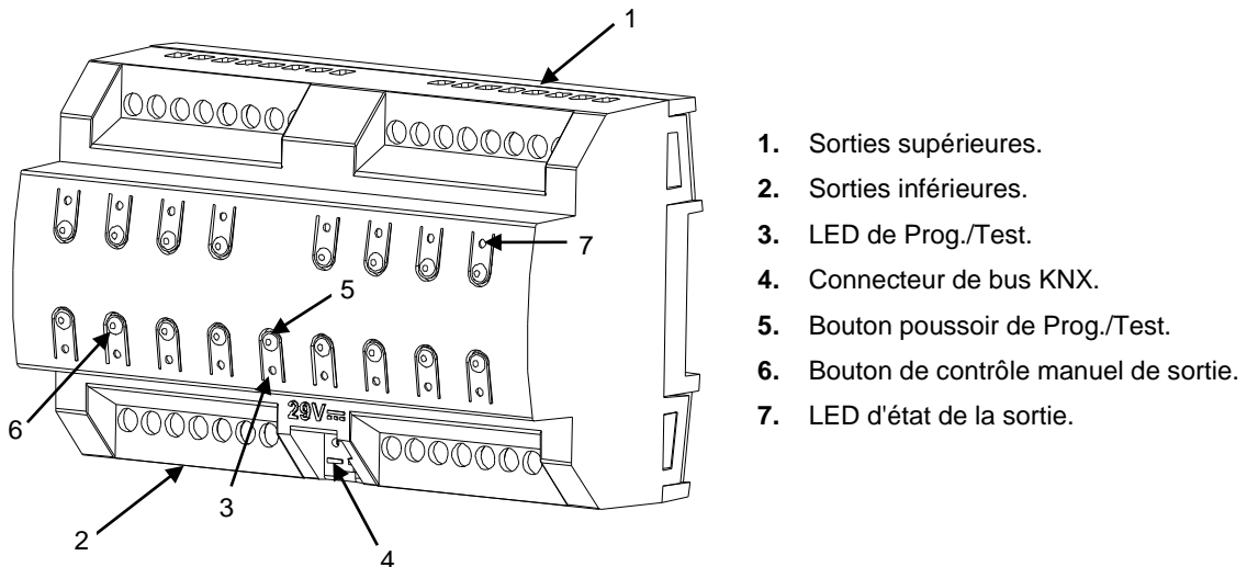
Figure 1. Diagramme des éléments du MAXinBOX 24.
