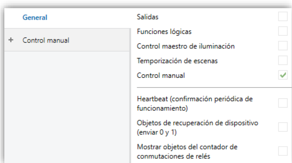
Figura 3. Pantalla general.
