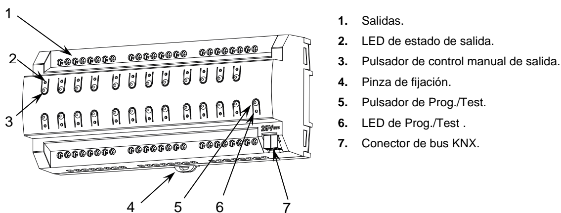
Figura 1. Diagrama de elementos del MAXinBOX 24 v2.
