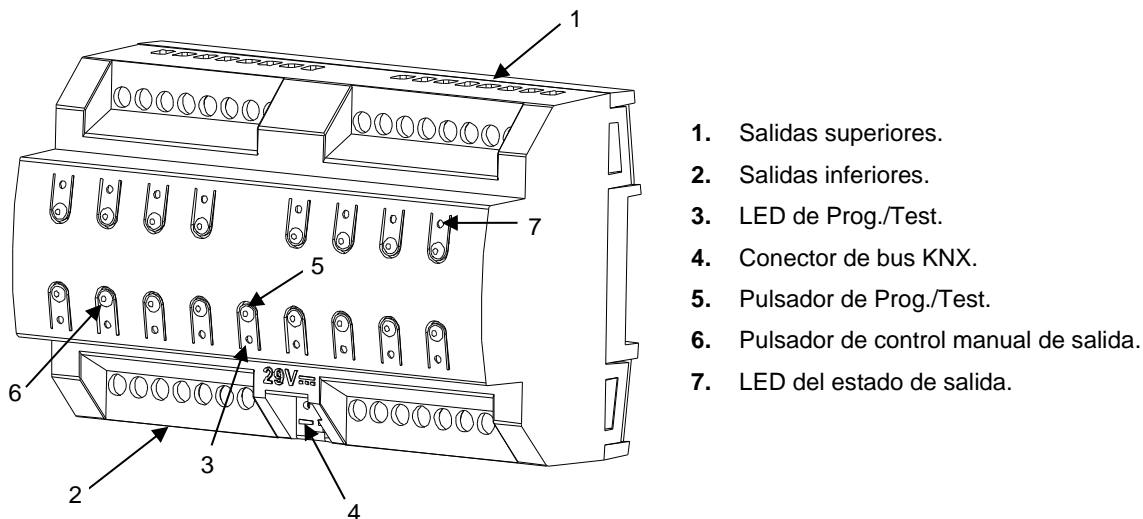
Figura 1. Diagrama de elementos del MAXinBOX 24 v2.
