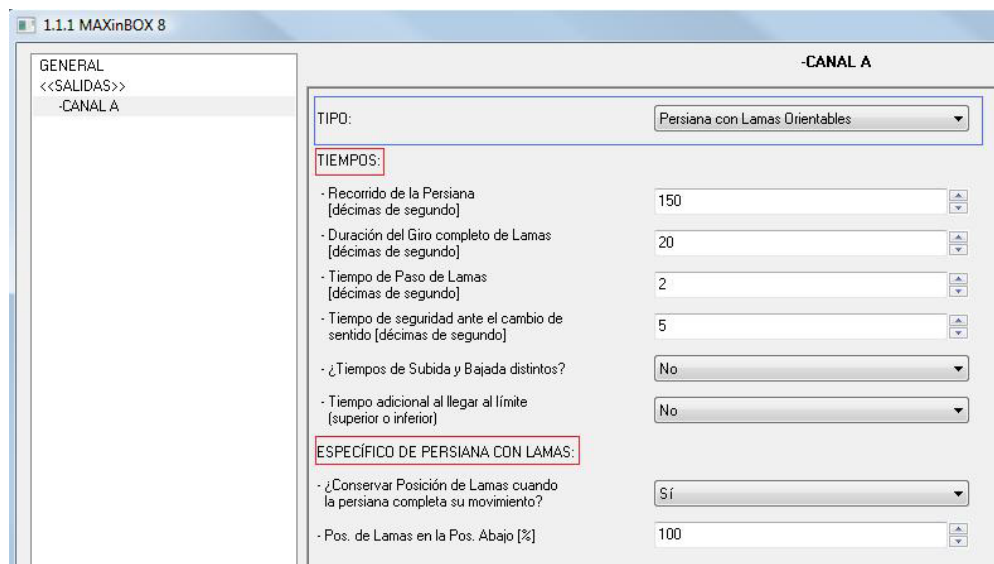
Figura 21. Configuración de persianas con lamas en ETS
