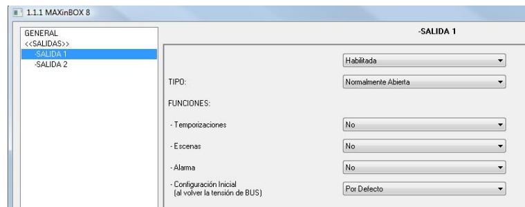
Figura 7. Canal A configurado como salidas individuales
