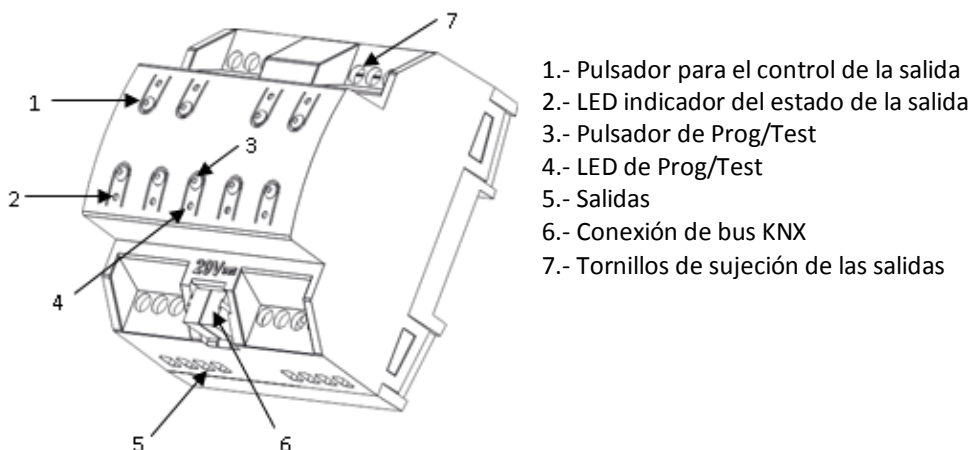
Figura 2. MAXinBOX 8. Esquema de elementos
