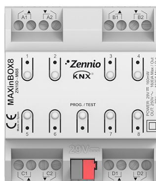
Figura 1. Actuador MAXinBOX 8
