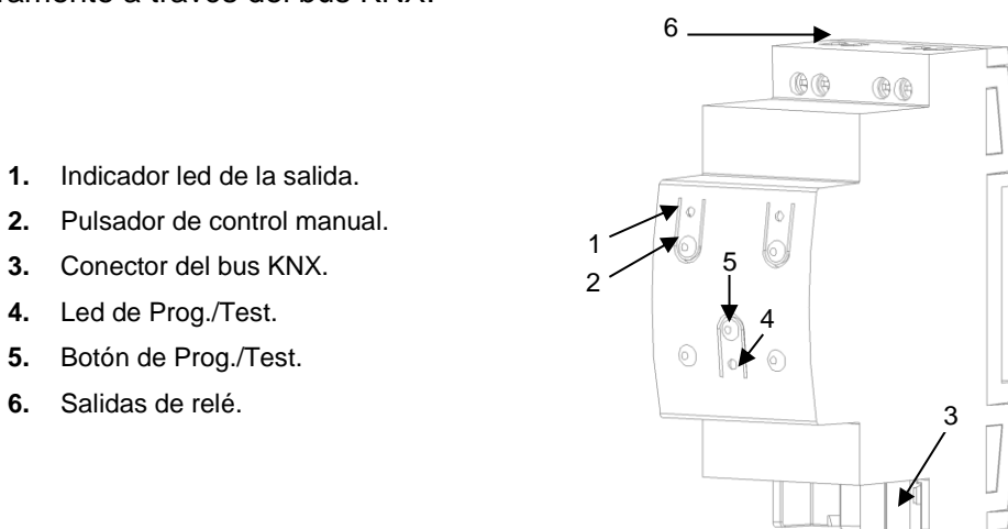
Figura 1. MINiBOX 20. Elementos.
