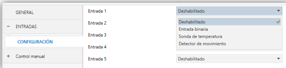
Figura 5 Entradas - Configuración.
