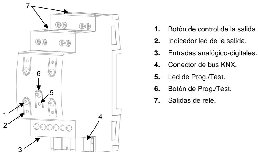
Figura 1. MINiBOX 45. Elementos.
