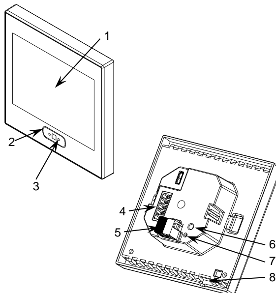
Figura 1. Diagrama de elementos Z35.
