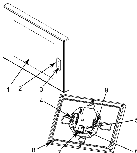
Figura 2. Diagrama de elementos Z40.
