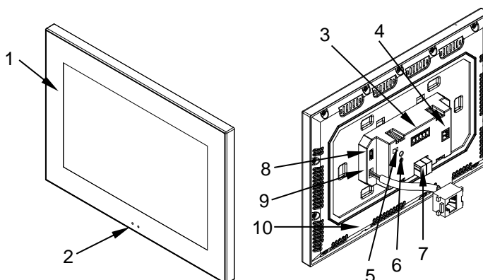
Figura 1 Diagrama de elementos.
