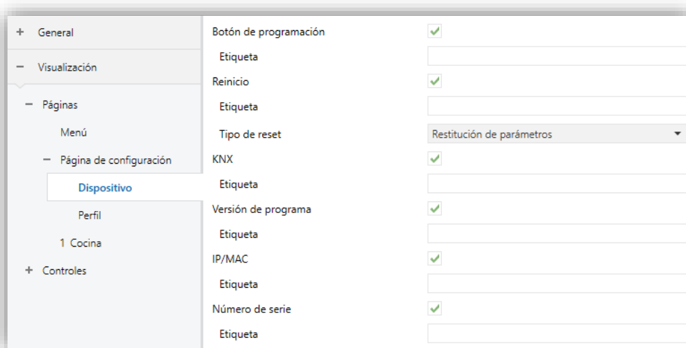
Figura 49. Página de configuración. Dispositivo.
