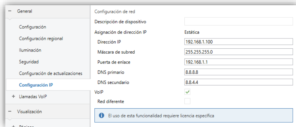
Figura 24. Configuración IP con VoIP habilitado en misma red
