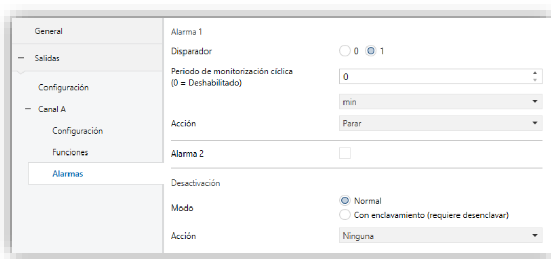
Figura 4. Canal persiana - Alarmas.
