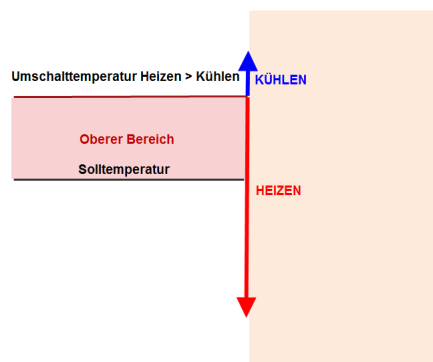
Bild 24. Umschalten Heizen auf Kühlen
