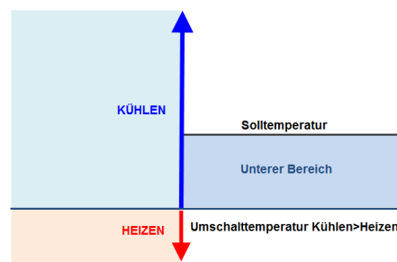
Bild 25. Umschalten Heizen auf Kühlen
