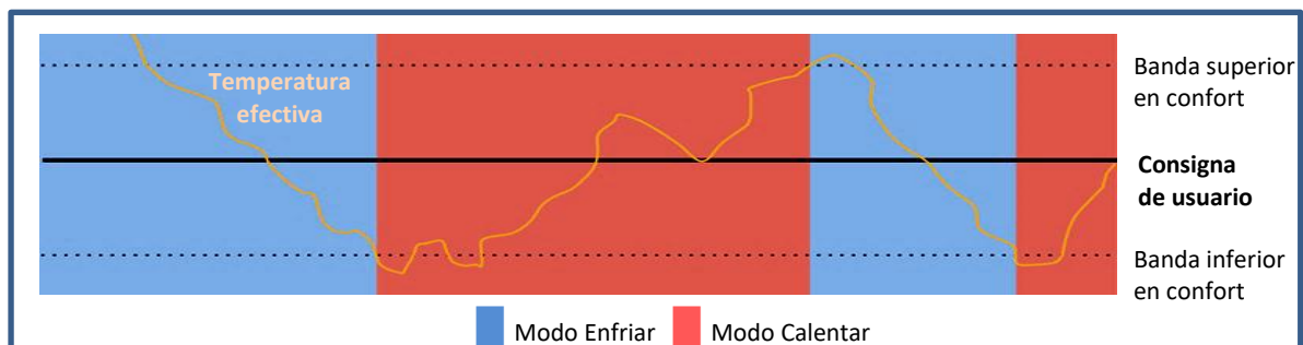
Figura 3. Cambio de modo automático en modo Confort.
