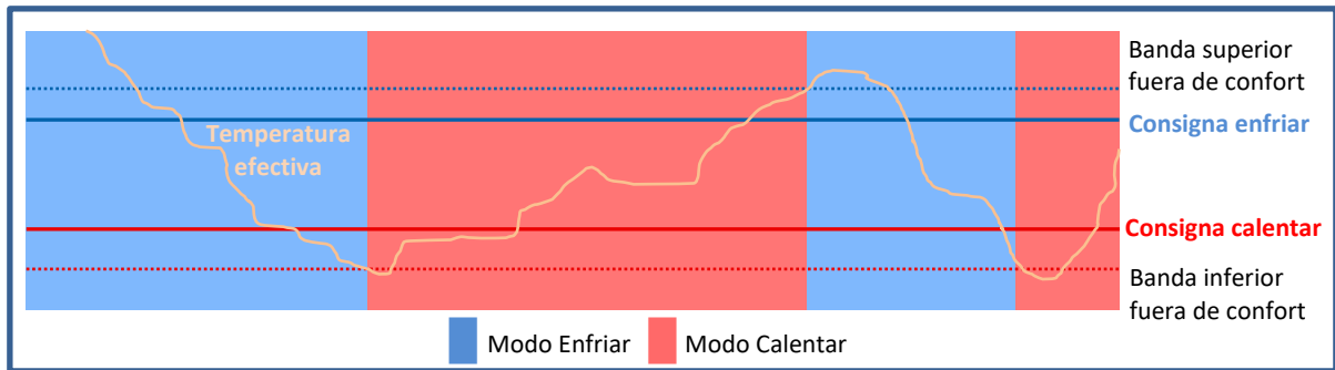
Figura 2. Cambio de modo automático en modos Standby , Económico y Protección.
