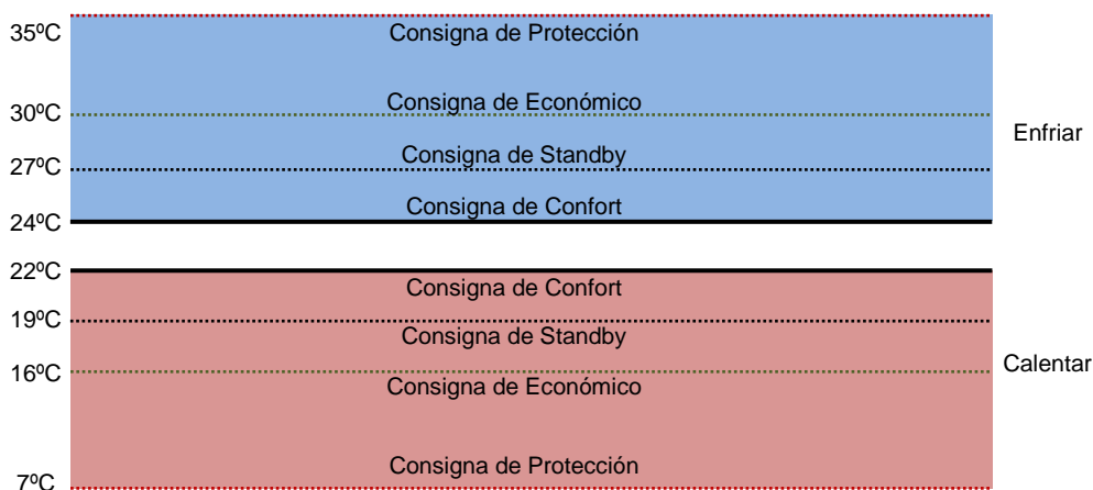
Figura 1. Consignas por defecto.
