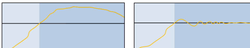
Figura 6. Efecto de reiniciar o no el error integral acumulado tras saturación.
