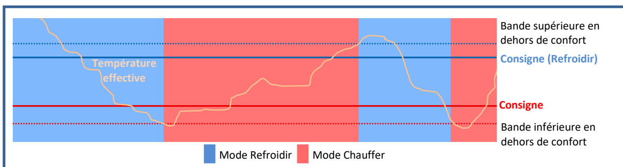
Figure 2. Changement de mode automatique à modes Veille, Économique et Protection .
