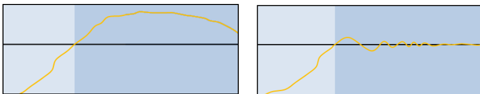
Figure 6. Effet de réinitialiser ou non l'erreur accumulée après saturation.
