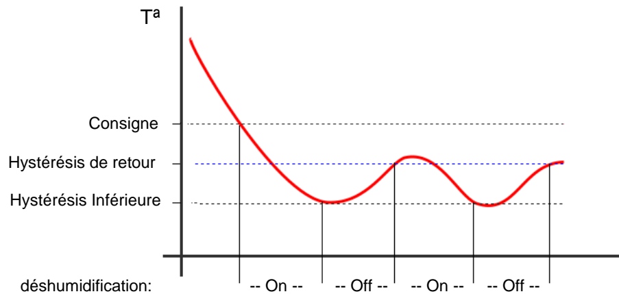
Figure 7. déshumidification: Hystérésis de retour
