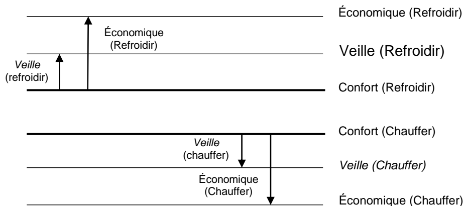
Figure 7. Diagramme de consignes absolues
