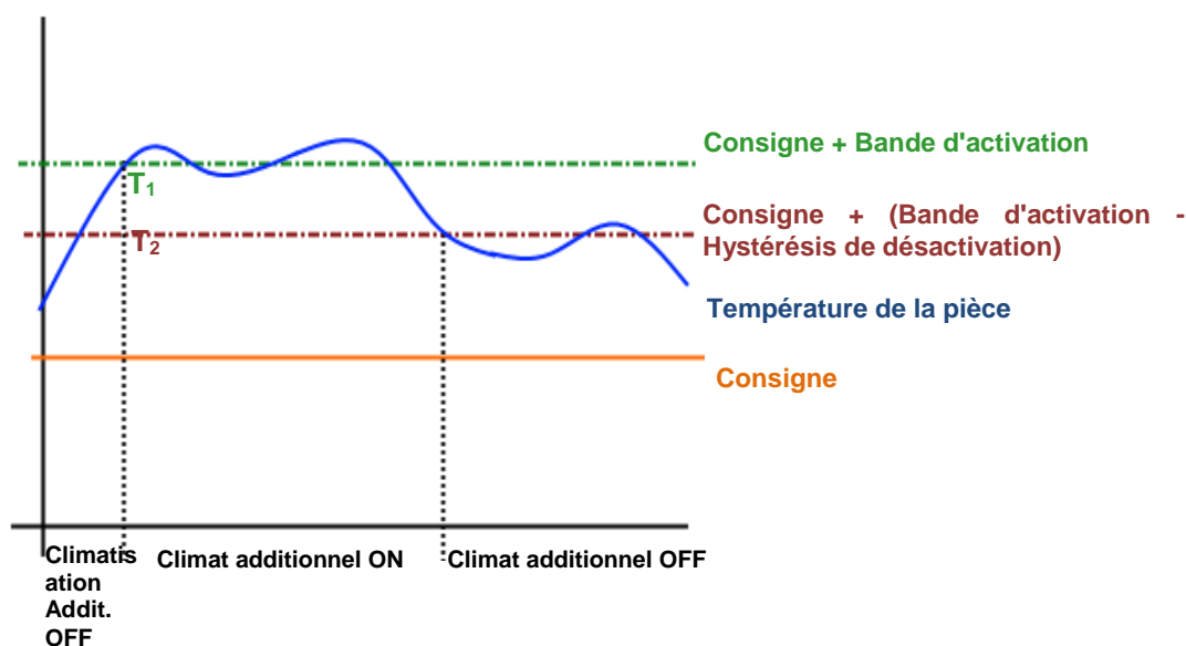
Figure 5. Activation et désactivation du système additionnel en mode refroidir.
